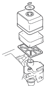
фильтрующий элемент
